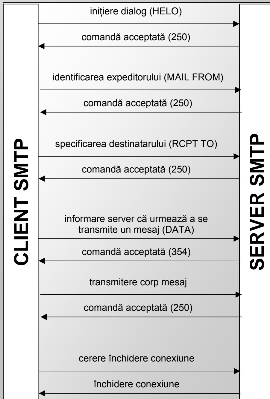
Diagrama 2.1.3 Dialogul SMTP pentru transferul unui mesaj de la procesul client către procesul server.
